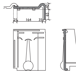
Tuile de rive droite
