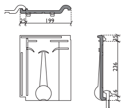
Demi tuile gauche
