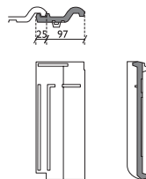
Tuile membron (pas de demi tuile membron)
