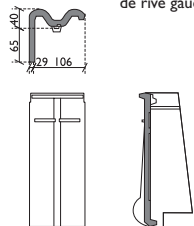
Demi tuile de rive gauche
