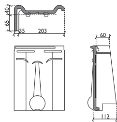
Demi tuile de rive gauche
